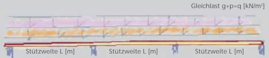
Dreifeldträger für g+p=q für L/400 tel ungünstig überlagert g/p = 0.5 bis 1.5
