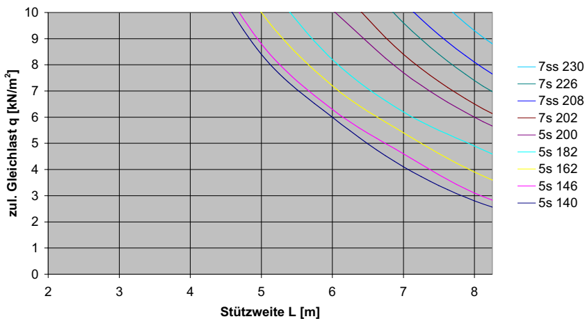
Zweifeldträger für Volllast für L/300 tel
