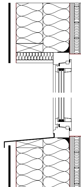
Abb. 17: Vertikalschnitt – Fensteranschluss mit Befestigungswinkel
