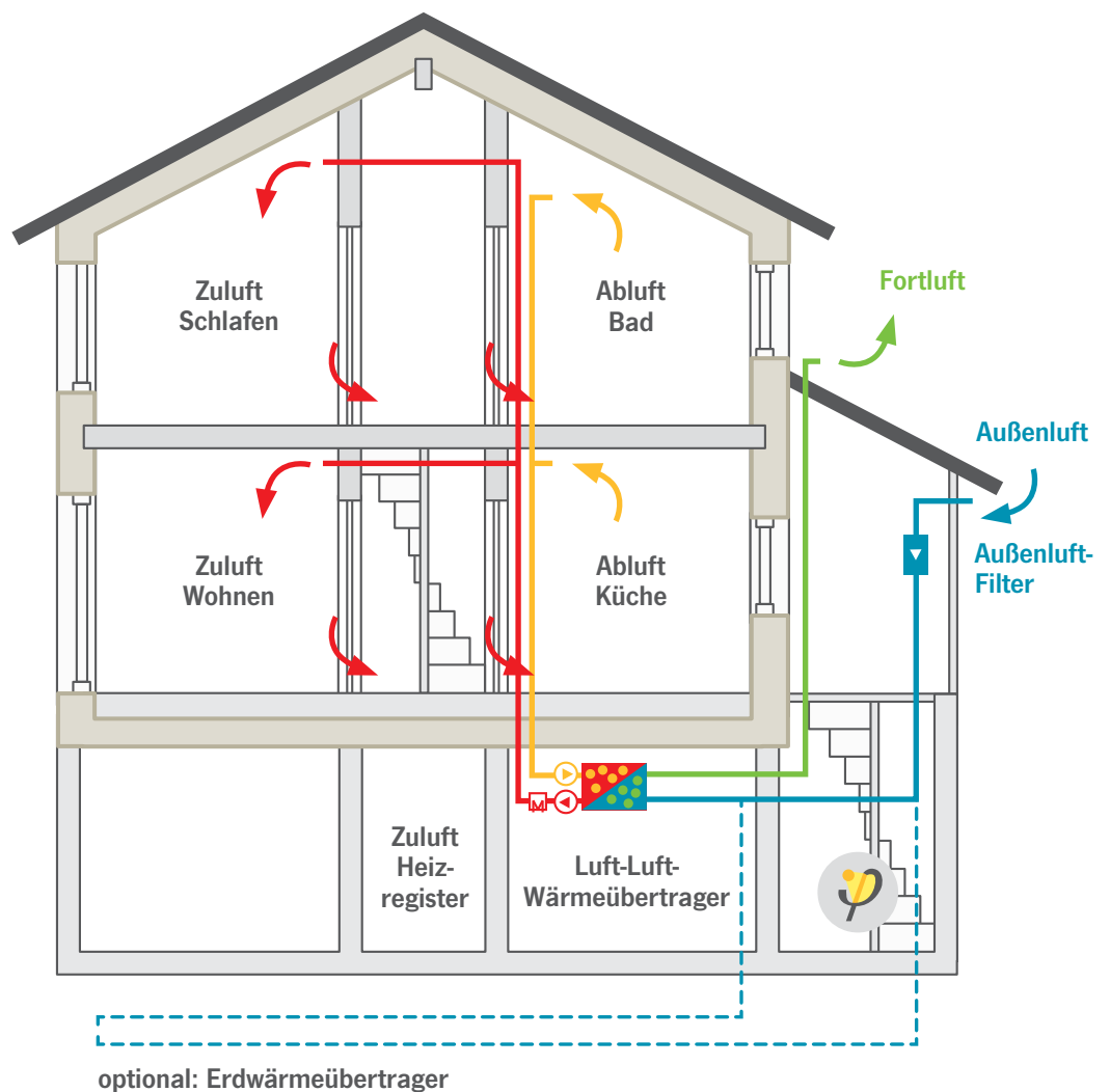
Abb. 12: Mit moderner Lüftungstechnologie kann mittlerweile das 8 bis 15-fache an Energie aus der Abluft zurückgehalten werden, als zu ihrem Betrieb notwendig ist.
